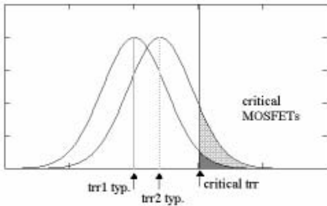
Fig. 9. Critical MOSFETs versus trr.
